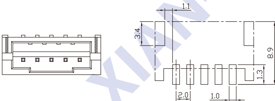
P.C.B LAYOUT
