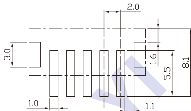
P.C.B LAYOUT
