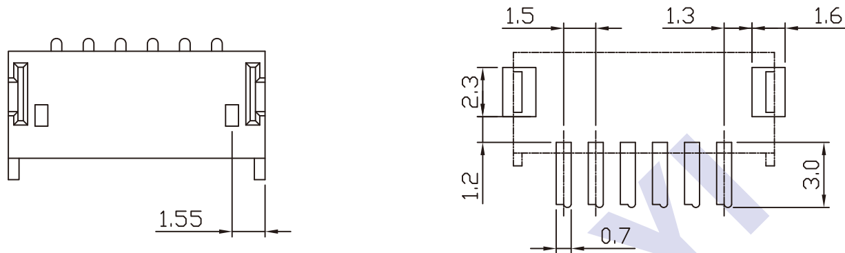
P.C.B LAYOUT
