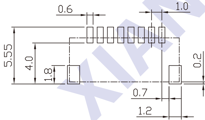
P.C.B LAYOUT
