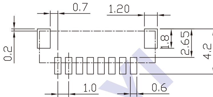
P.C.B LAYOUT
